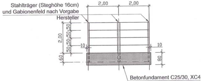
Ansicht RQ3/ Fundament C/ Stützenabstand 2,00m
