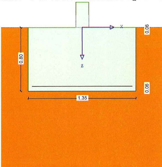
Ansicht RQ2/ Fundament B/ Stützenabstand 2,00m
