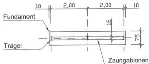
Draufsicht RQ3/ Fundament C/ Stützenabstand 2,00m
