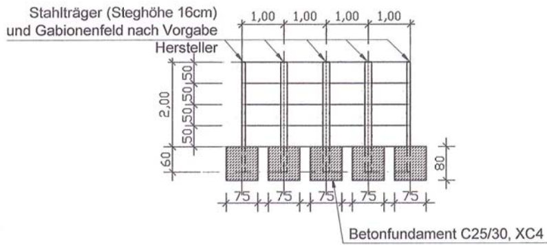
Ansicht RQ4/ Fundament A/ Stützenabstand 1,00m
