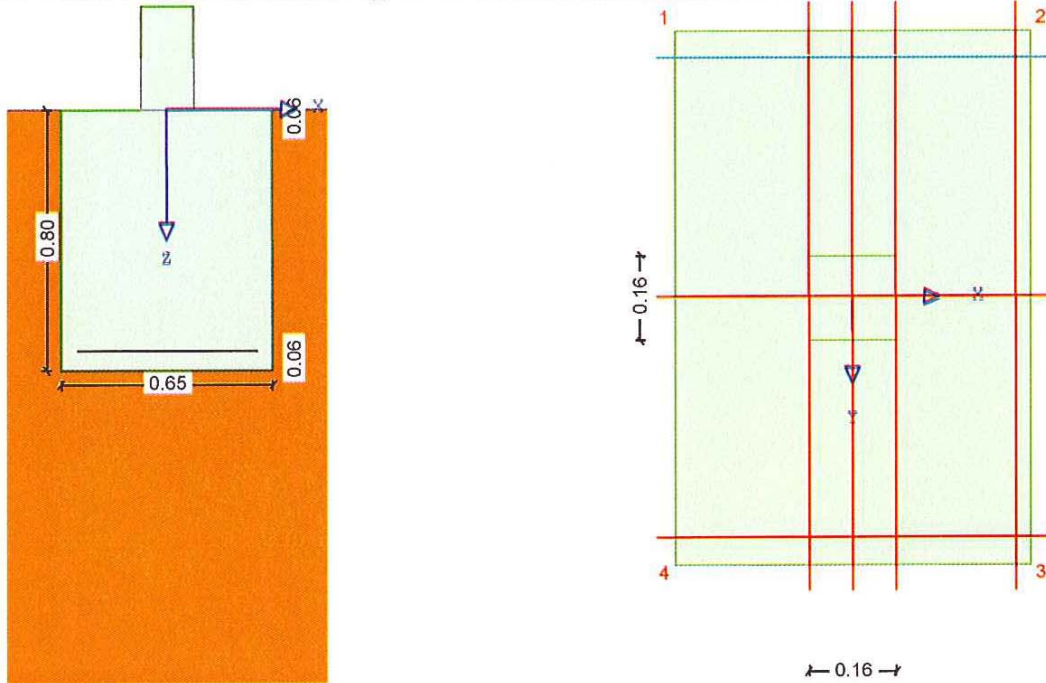
Ansicht RQ6/ Fundament C/ Stützenabstand 1,00m
