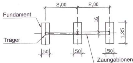
Draufsicht RQ2/ Fundament B/ Stützenabstand 2,00m
