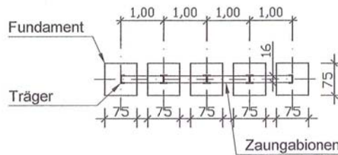
Draufsicht RQ4/ Fundament A/ Stützenabstand 1,00m
