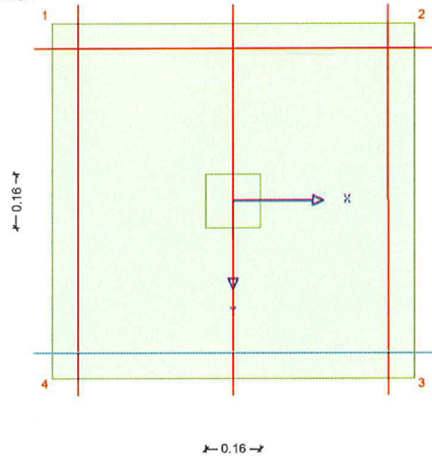
Ansicht RQ1/ Fundament A/ Stützenabstand 2,00m
