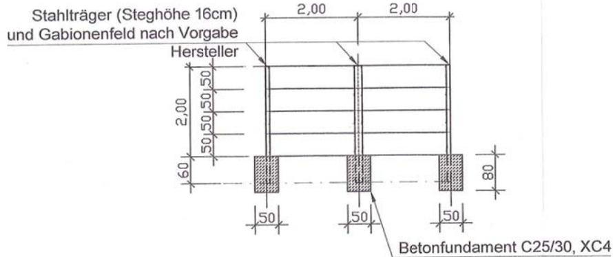
Ansicht RQ2/ Fundament B/ Stützenabstand 2,00m
