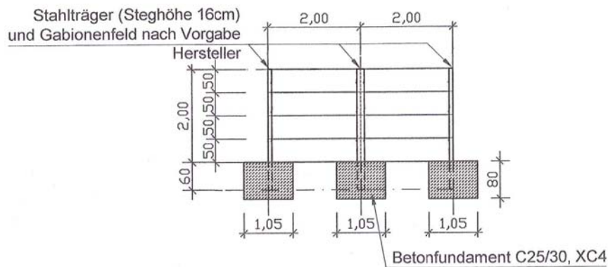
Ansicht RQ1/ Fundament A/ Stützenabstand 2,00m
