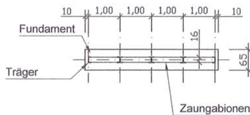
Draufsicht RQ6/ Fundament C/ Stützenabstand 1,00m
