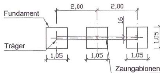
Draufsicht RQ1/ Fundament A/ Stützenabstand 2,00m
