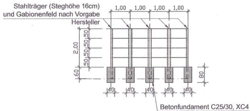
Ansicht RQ5/ Fundament B/ Stützenabstand 1,00m
