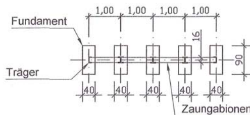
Draufsicht RQ5/ Fundament B/ Stützenabstand 1,00m
