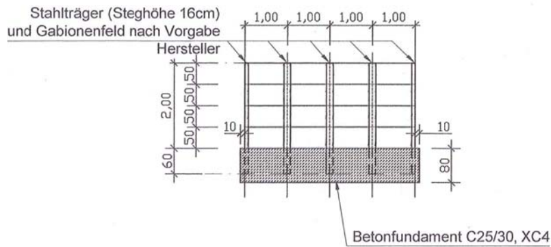
Ansicht RQ6/ Fundament C/ Stützenabstand 1,00m
